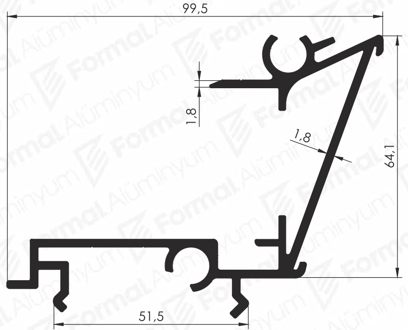
Pr.No: 9210 1,529 kg/m
