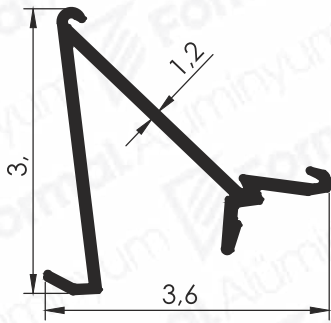
Pr.No: 9245 0,340 kg/m
