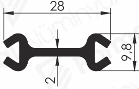
Pr.No: 9850 0,274 kg/m
