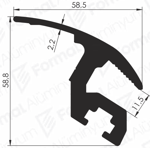
Pr.No: 941 1,911 kg/m
