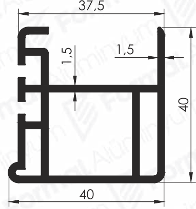
Pr.No: 9521 0,861 kg/m
