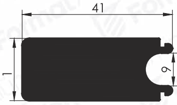
Pr.No: 9225 1,684 kg/m
