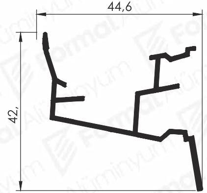
Pr.No: 9244 0,436 kg/m
