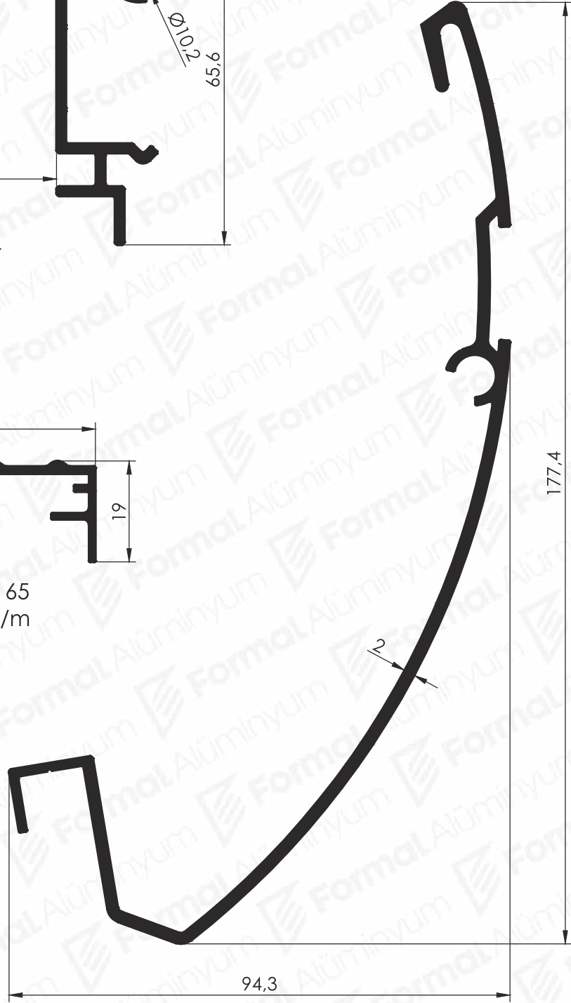
Pr.No: 9164 1,298 kg/m
