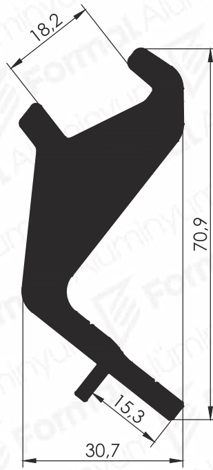
Pr.No: 9216 2,379 kg/m
