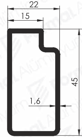
Pr.No: 9523 0,538 kg/m
