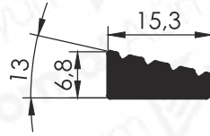
Pr.No: 9452 0,201 kg/m
