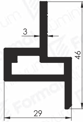
Pr.No: 9321 0,808 kg/m
