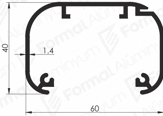
Pr.No: 9673 0,695 kg/m
