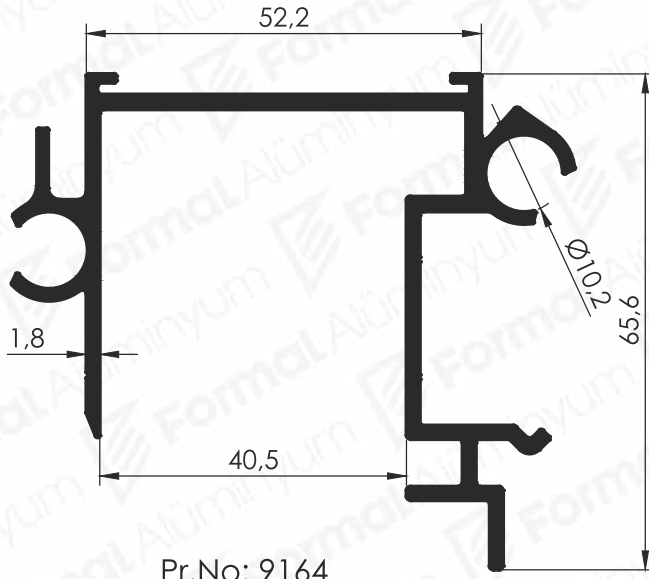
Pr.No: 9164 1,298 kg/m
