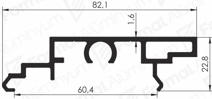
Pr.No: 9463 0,786 kg/m
