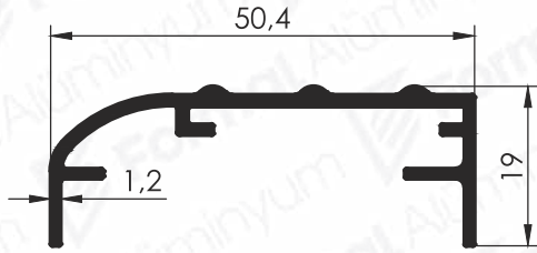
Pr.No: 9165 0,374 kg/m
