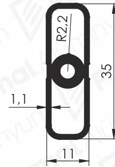
Pr.No: 9524 0,349 kg/m
