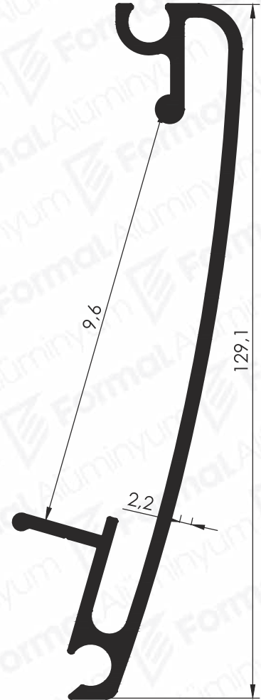
Pr.No: 9464 1,402 kg/m
