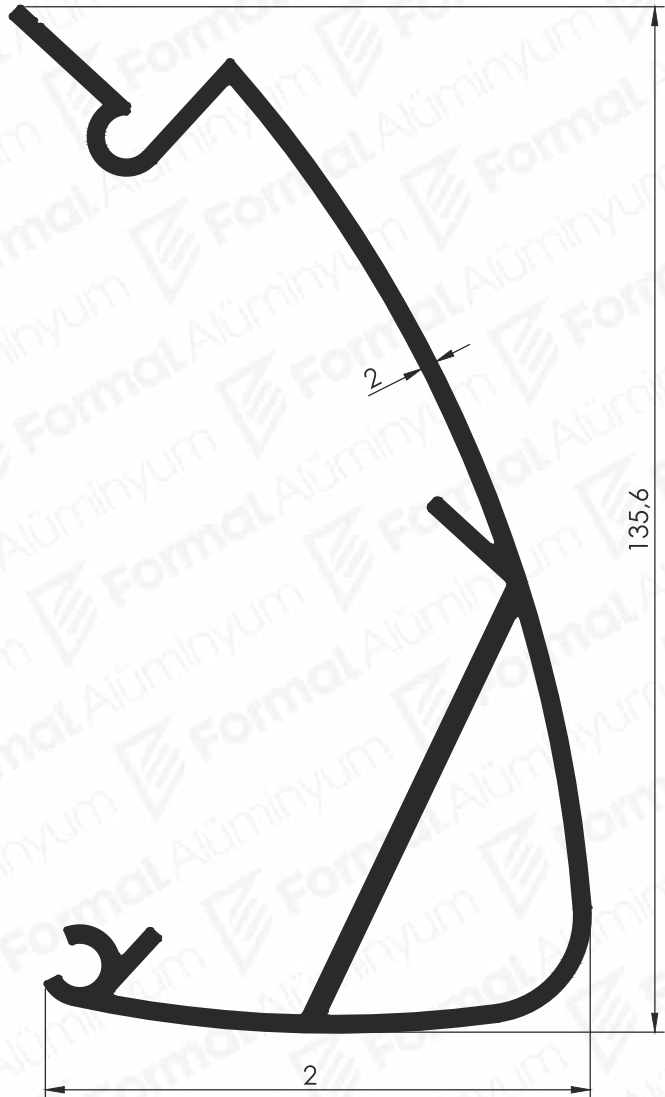
Pr.No: 9224 1,963 kg/m
