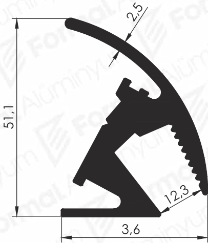
Pr.No: 9181 1,529 kg/m
