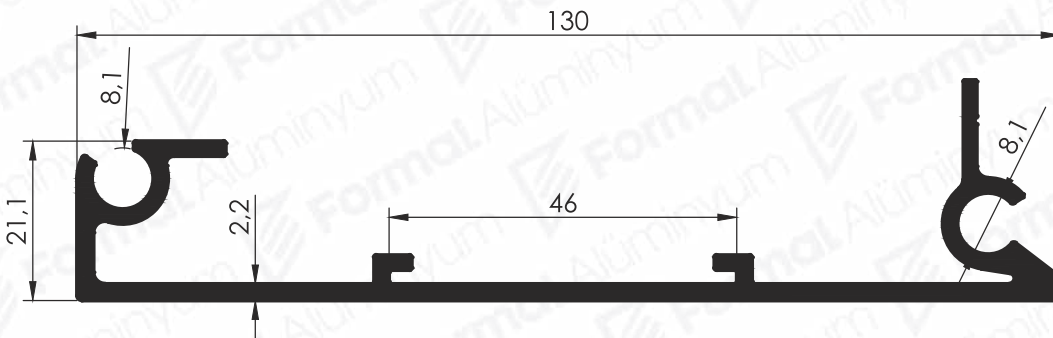
Pr.No: 9319 1,358 kg/m
