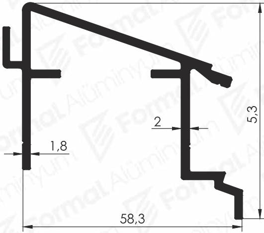
Pr.No: 9219 0,93 kg/m
