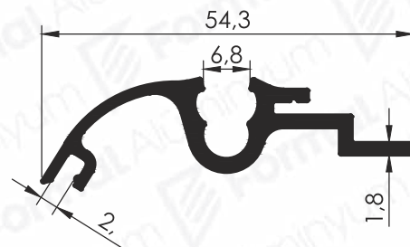
Pr.No: 9283 0,458 kg/m
