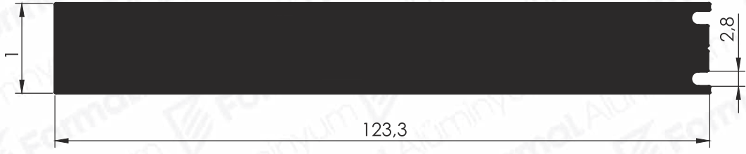
Pr.No: 9415 5,622 kg/m
