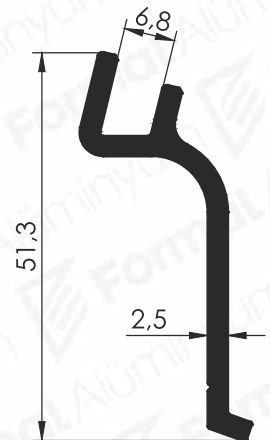
Pr.No: 9217 0,492 kg/m
