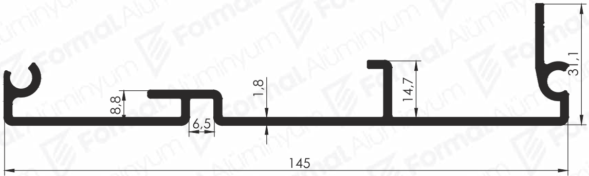
Pr.No: 9205 1,213 kg/m
