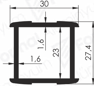
Pr.No: 9522 0,487 kg/m
