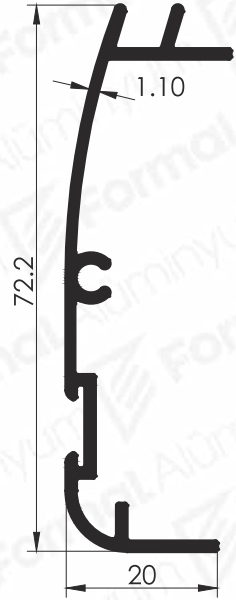
Pr.No: 9672 0,453 kg/m
