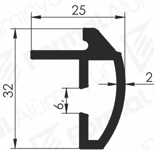
Pr.No: 9183 0,45 kg/m
