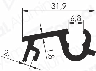
Pr.No: 9220 0,344 kg/m
