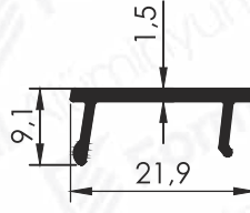
Pr.No: 9243 0,130 kg/m
