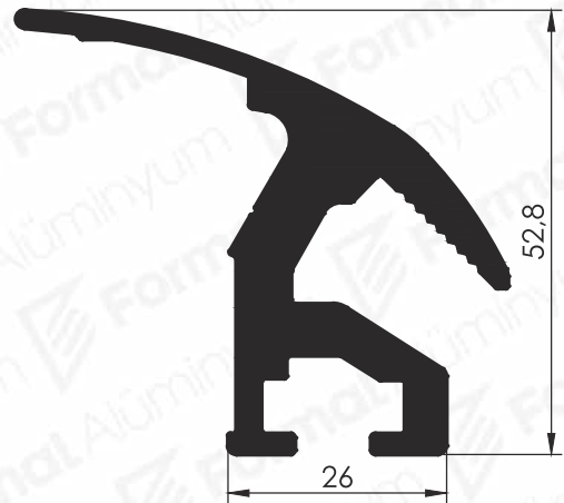
Pr.No: 931 1,814 kg/m
