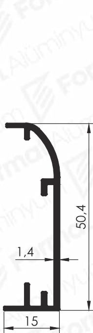
Pr.No: 9211 0,313 kg/m
