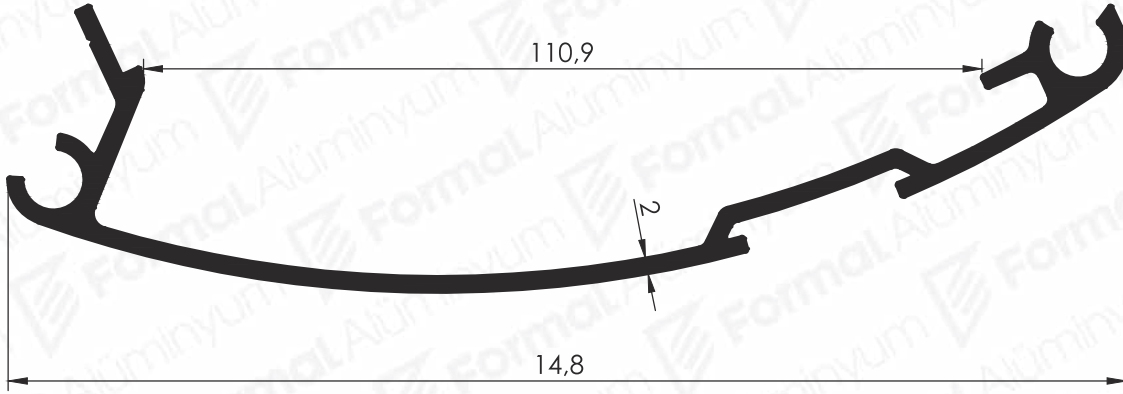
Pr.No: 9218 1,308 kg/m
